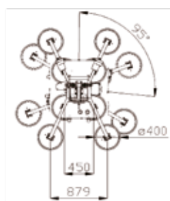
Drehposition
